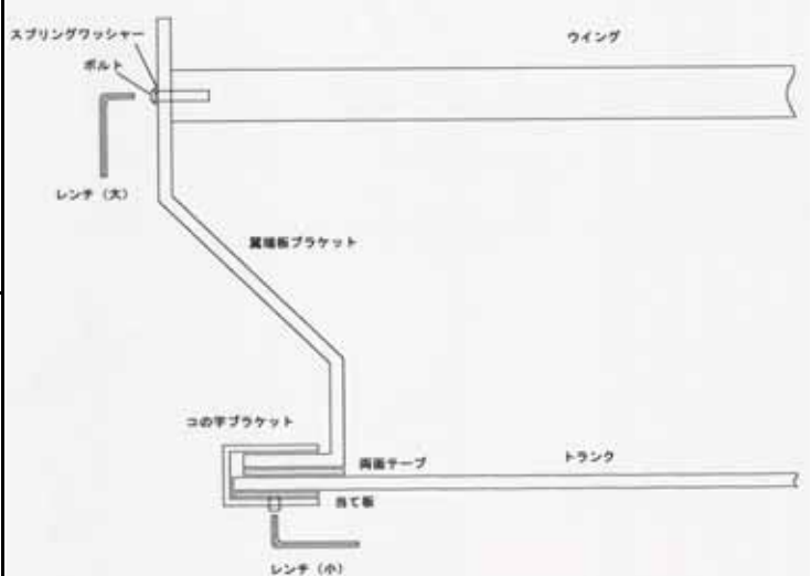
完成図
