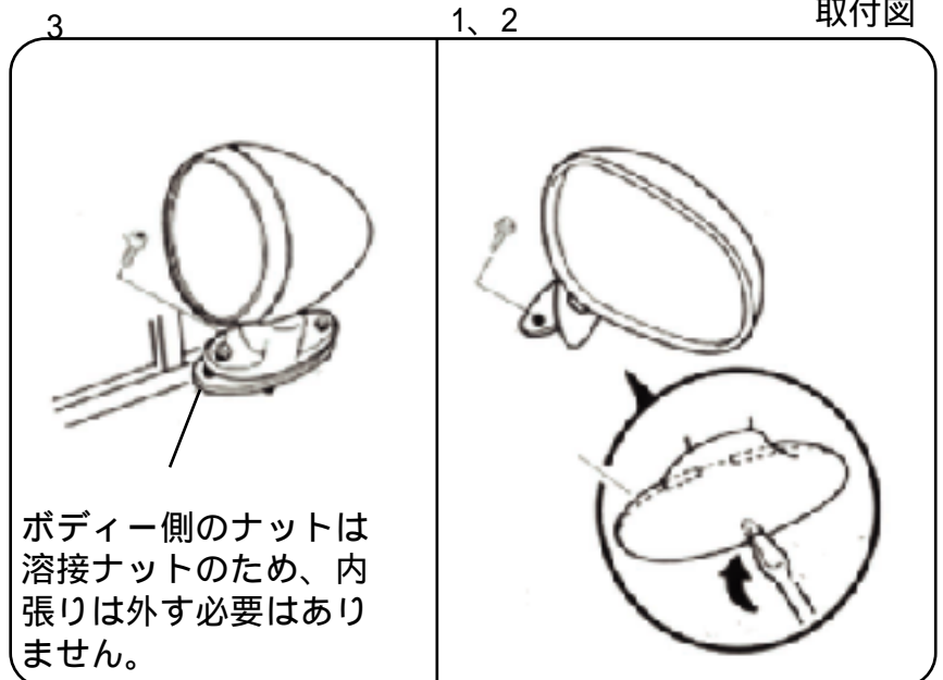
取付図
